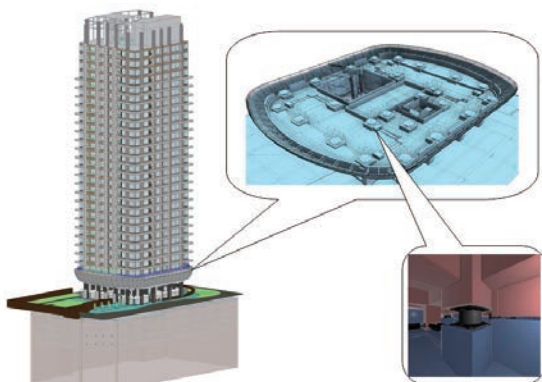
隔震层配置图
